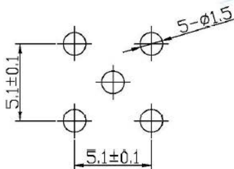
PCB建议安装板
