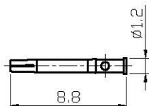
Pin contact中心针
